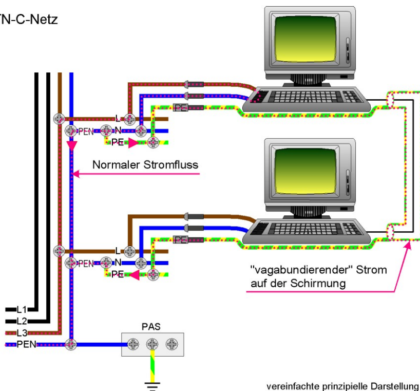
Abbildung 1: Entstehung von Ausgleichsströmen auf Schirmungen und die möglichen Gegenmaßnahmen bei einem TN-C-Netz
