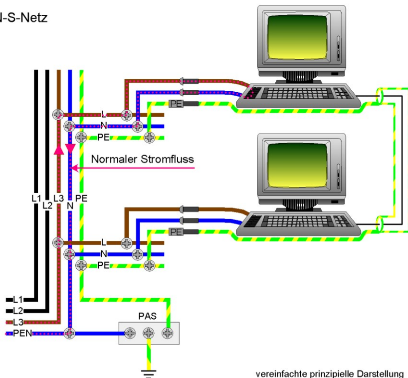
Abbildung 2: Entstehung von Ausgleichsströmen auf Schirmungen und die möglichen Gegenmaßnahmen bei einem TN-S-Netz
