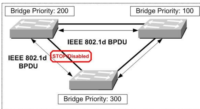
Abbildung 1: Spanning Tree
