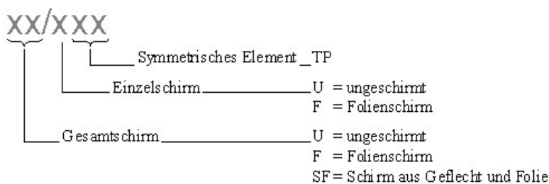
Abbildung 1: Systematik der Typbezeichnung von Kupferkabeln
